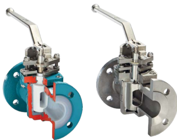
Prozess-Armaturen
